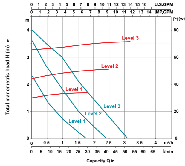
LRP25-40/130 — Q-H — Q-P
