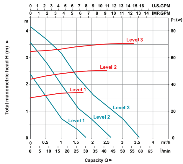
LRP25-40/180 — Q-H — Q-P
