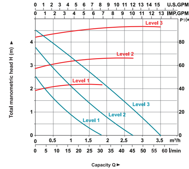
LRP21-50F/120 — Q-H — Q-P
