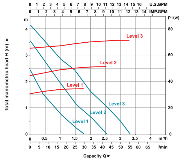
LRP21-40F/120 — Q-H — Q-P
