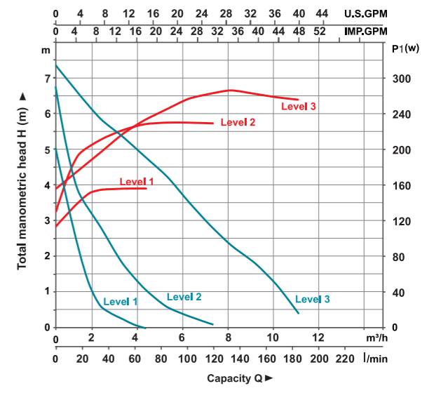
LRP32-80/180 LRP32-80F/220 LRP36-80F/200 LRP40-80F/250 — Q-H — Q-P
