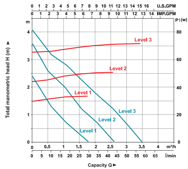
LRP32-40/180 — Q-H — Q-P
