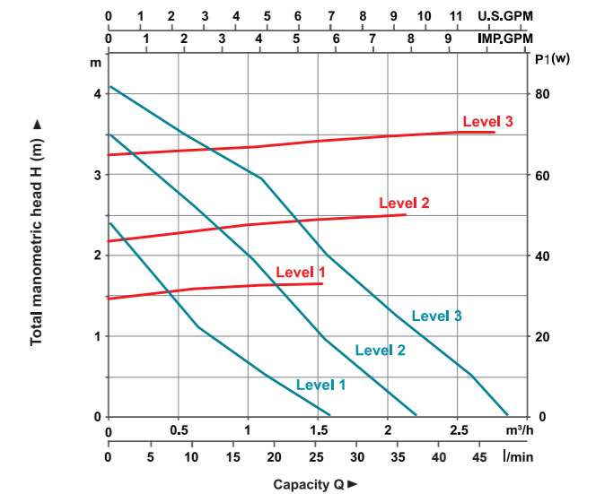
LRP20-40/130 — Q-H — Q-P
